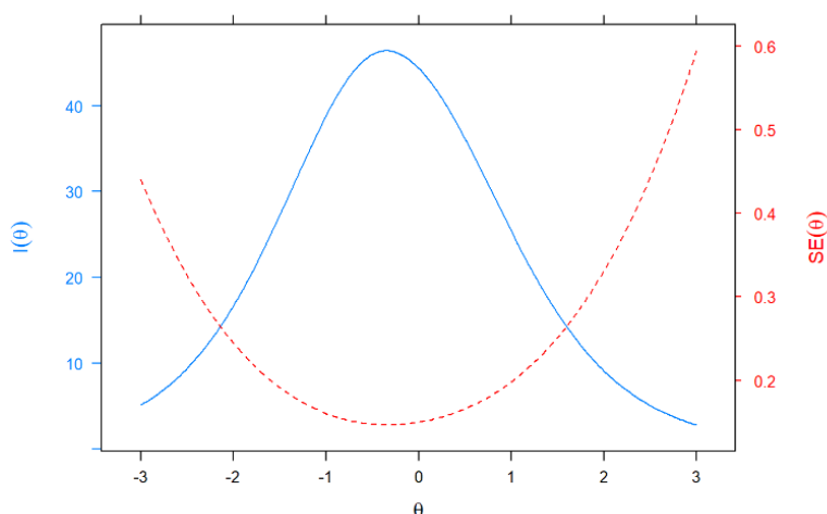
Figur 3. Testinformasjon og standard måle(u)sikkerheit 2023
