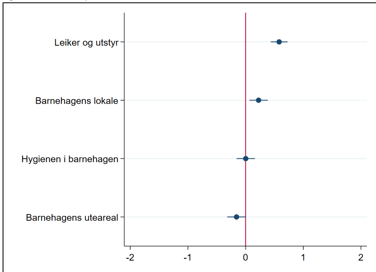
Figur A.1: Koeffisientplott, tilfredsheitsvariablar
